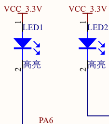
LED灯控制电路
