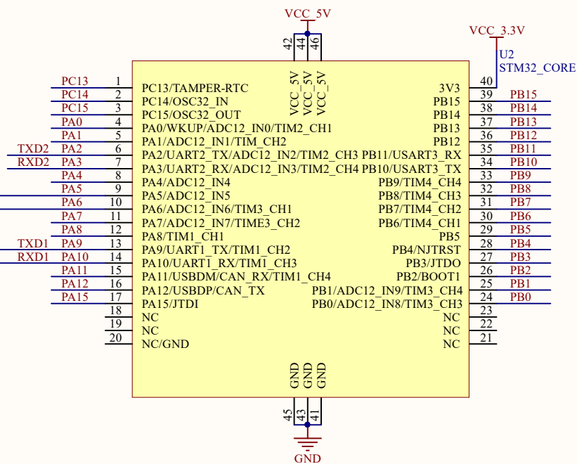
单片机核心板电路
